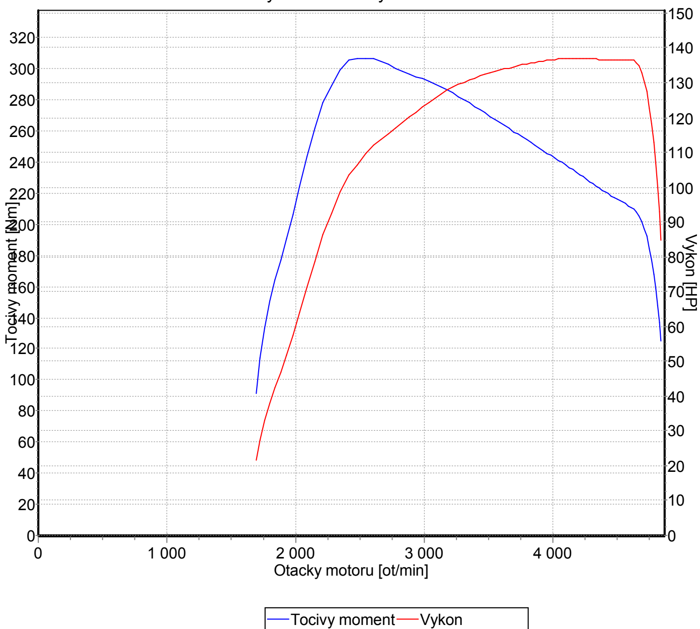
Tocivy moment a vykon motoru
